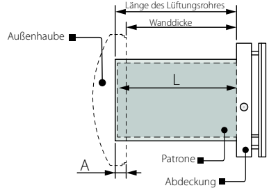
Wanddicke entspricht dem Minimalwert
