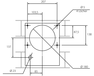
Markierung der Befestigungslöcher (mm)
