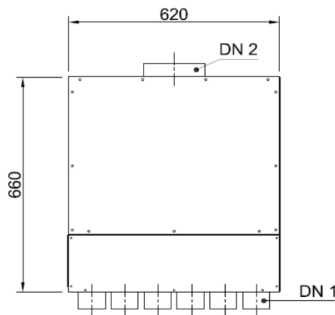
Draufsicht
